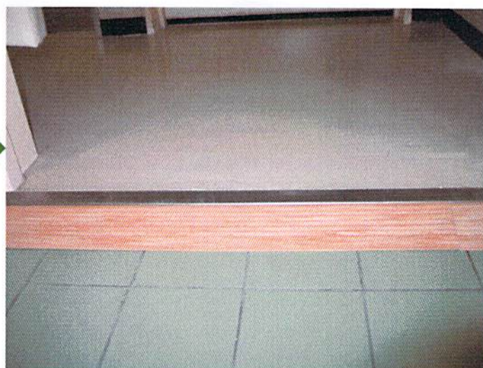
入口段差解消 (H100)
